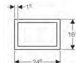
Geberit Sigma60, placca di comando Art. 115.792.GH.1
